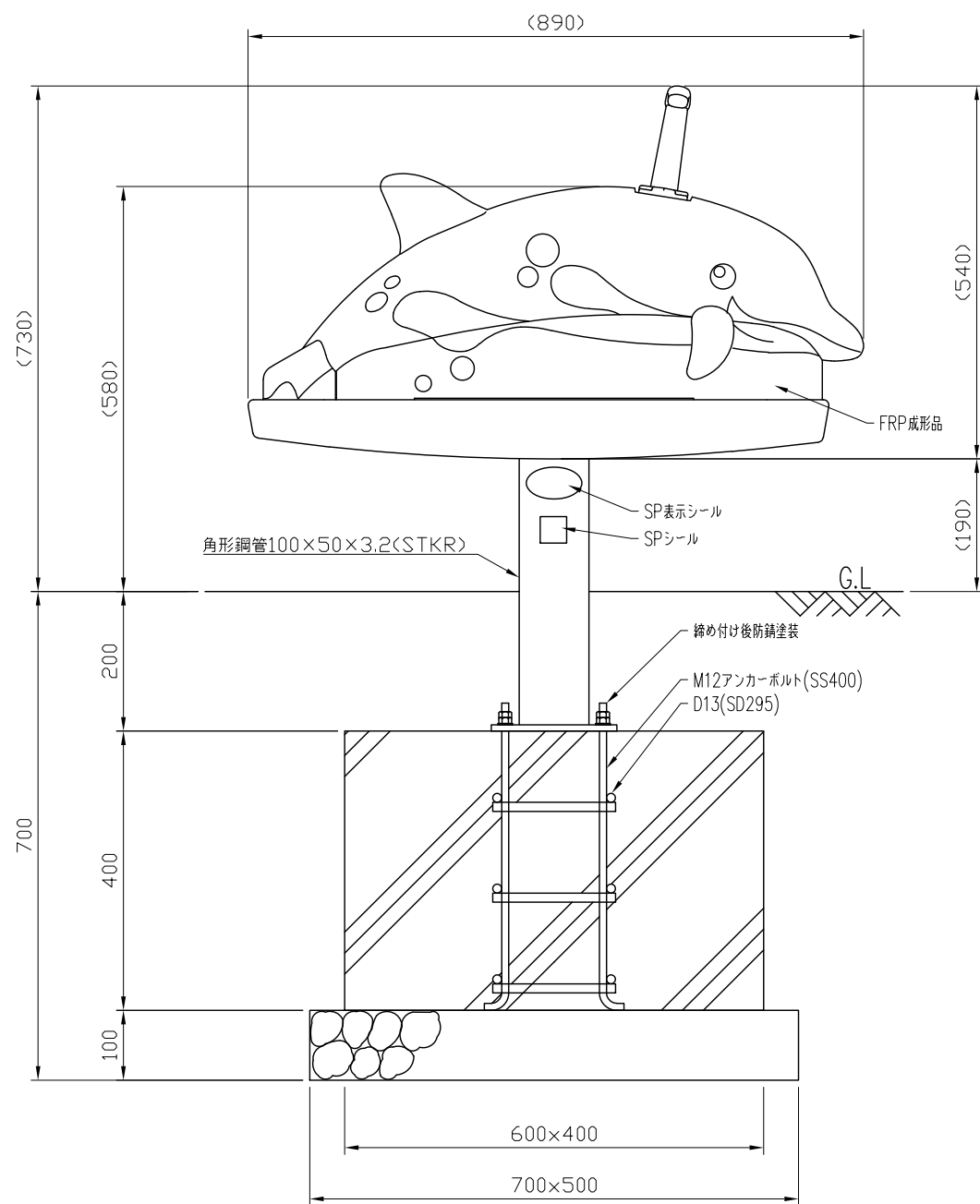
立面図 S=1:10
