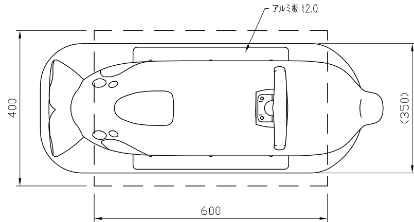
平面図 S=1:10
