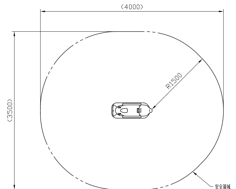
安全領域平面図 S=1:50
