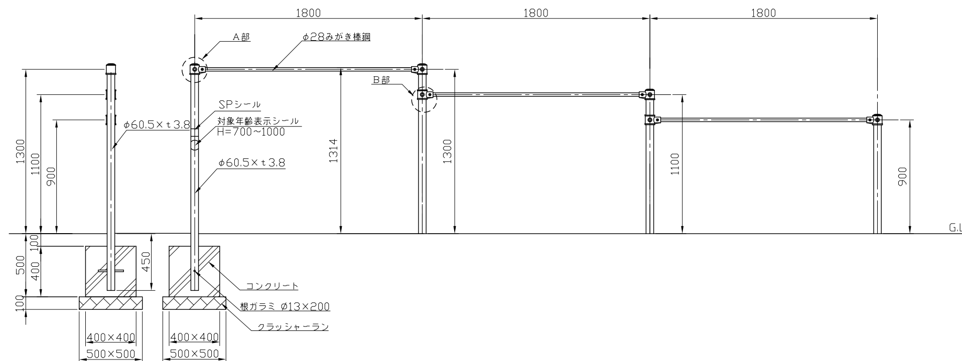
側面図 S=1:30
