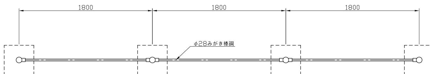
平面図 S=1:30
