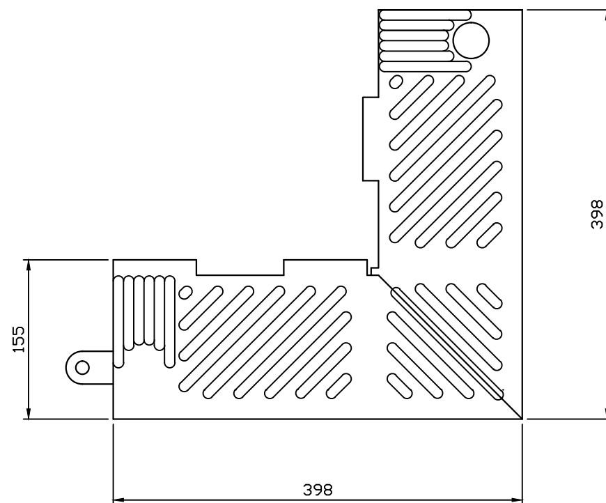
TSX455 スロープエッジコーナー
