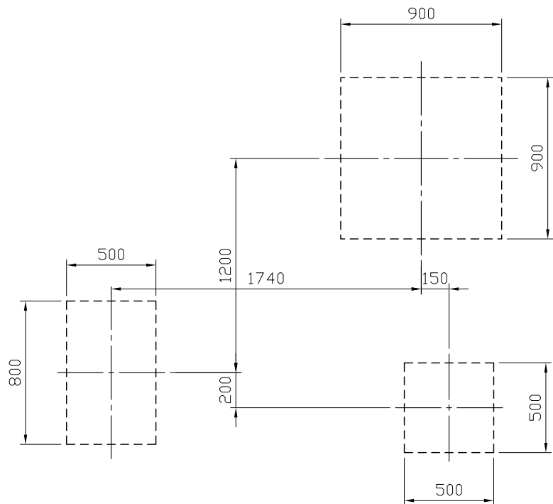
基礎伏図 S=1:30
