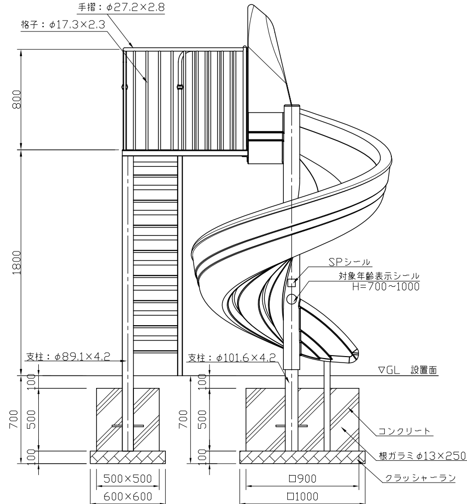
側面図 S=1:30
