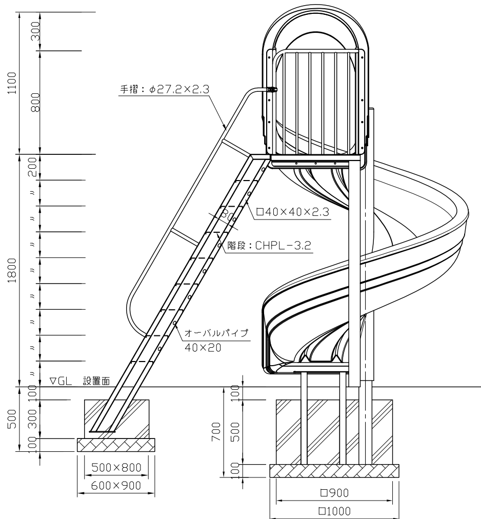
正面図 S=1:30
