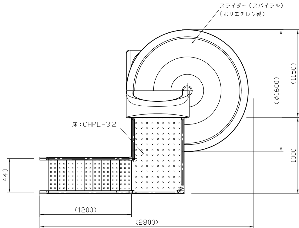
平面図 S=1:30
