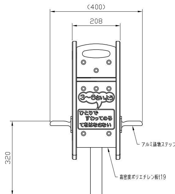
側面図 S=1:10
