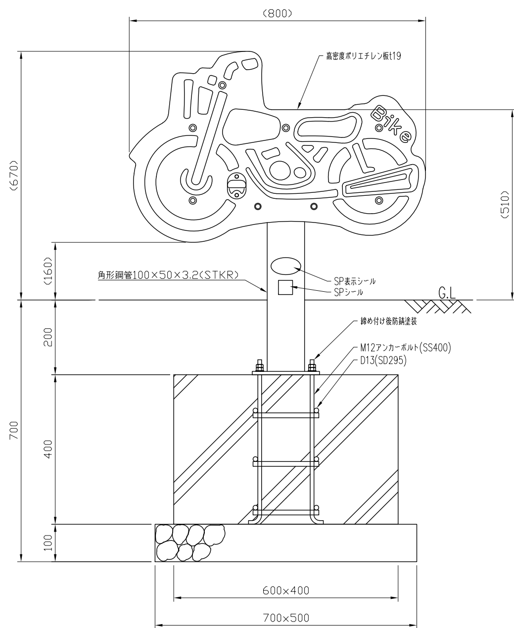
立面図 S=1:10
