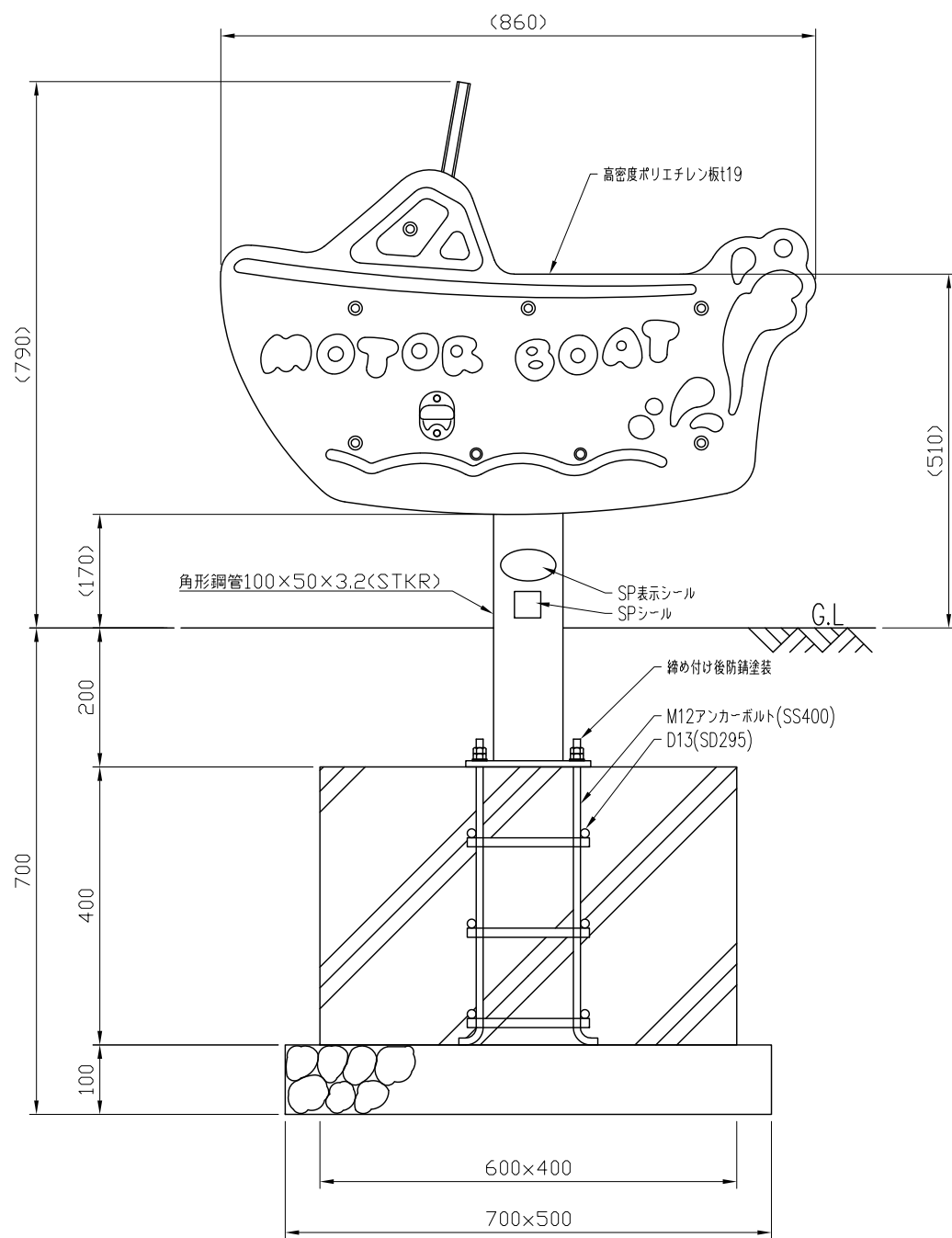
立面図 S=1:10
