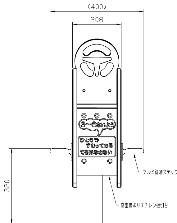
側面図 S=1:10
