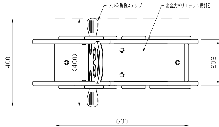
平面図 S=1:10
