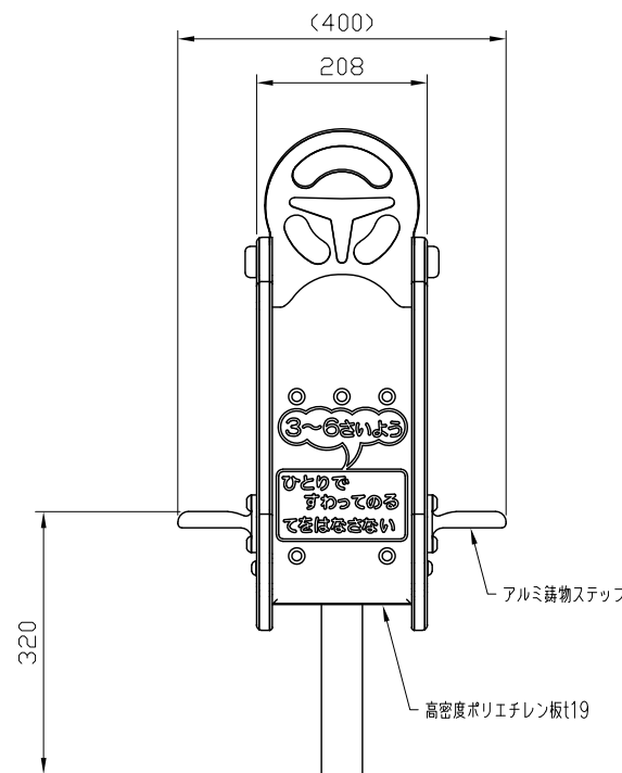
側面図 S=1:10
