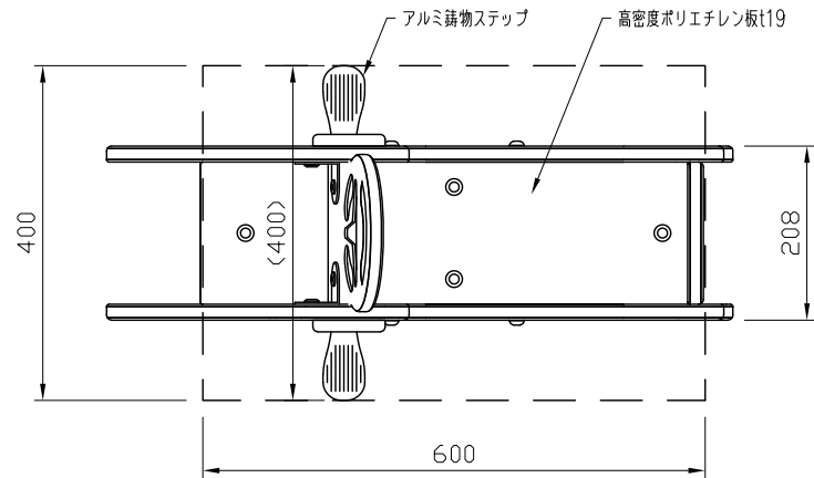
平面図 S=1:10
