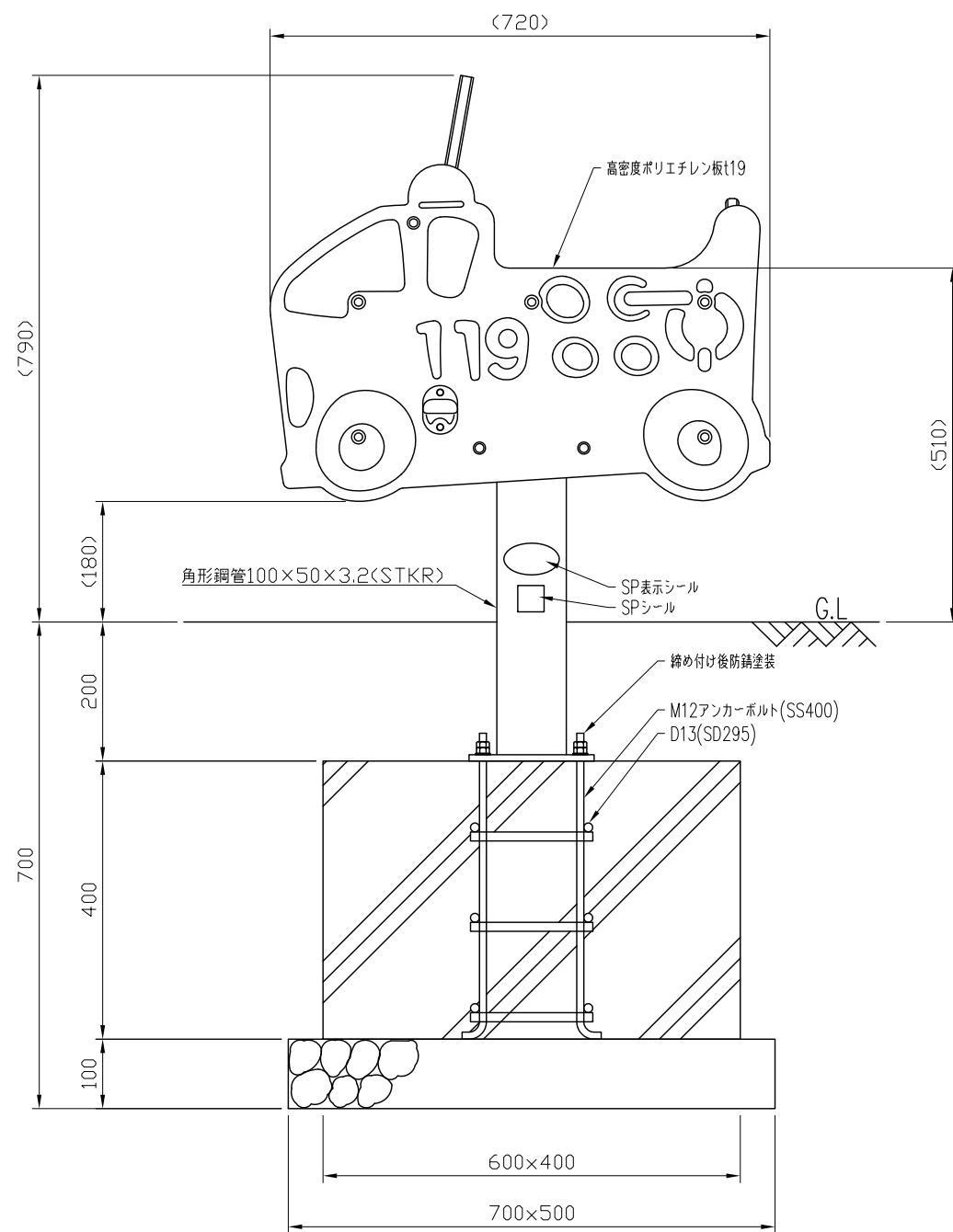
立面図 S=1:10
