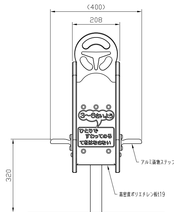
側面図 S=1:10
