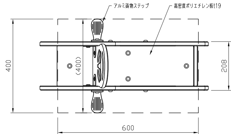
平面図 S=1:10
