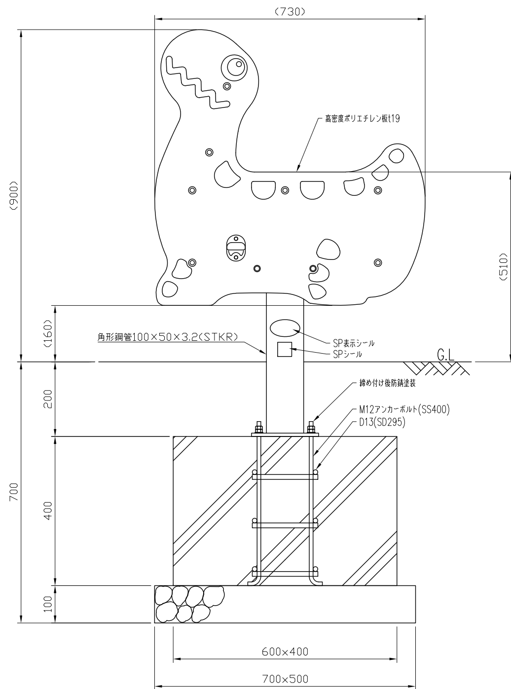
立面図 S=1:10
