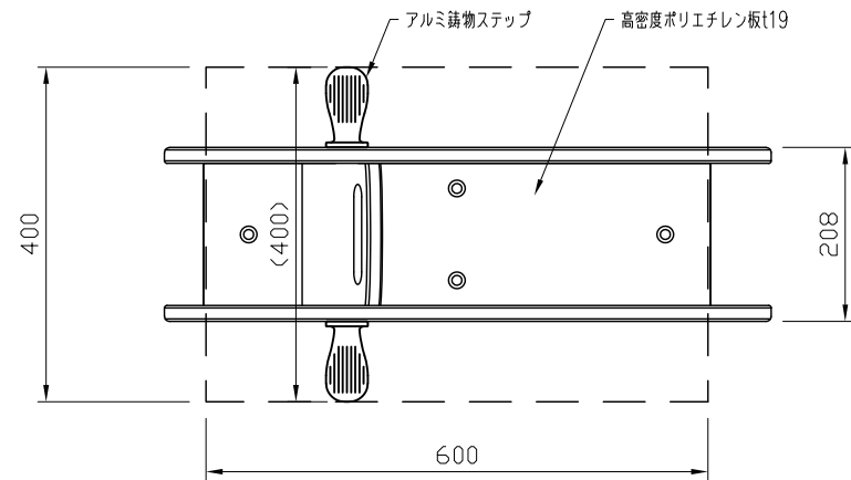
平面図 S=1:10
