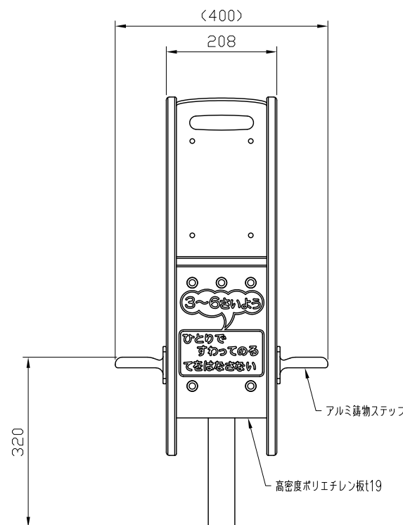
側面図 S=1:10
