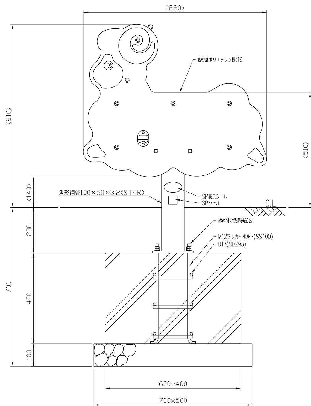
立面図 S=1:10
