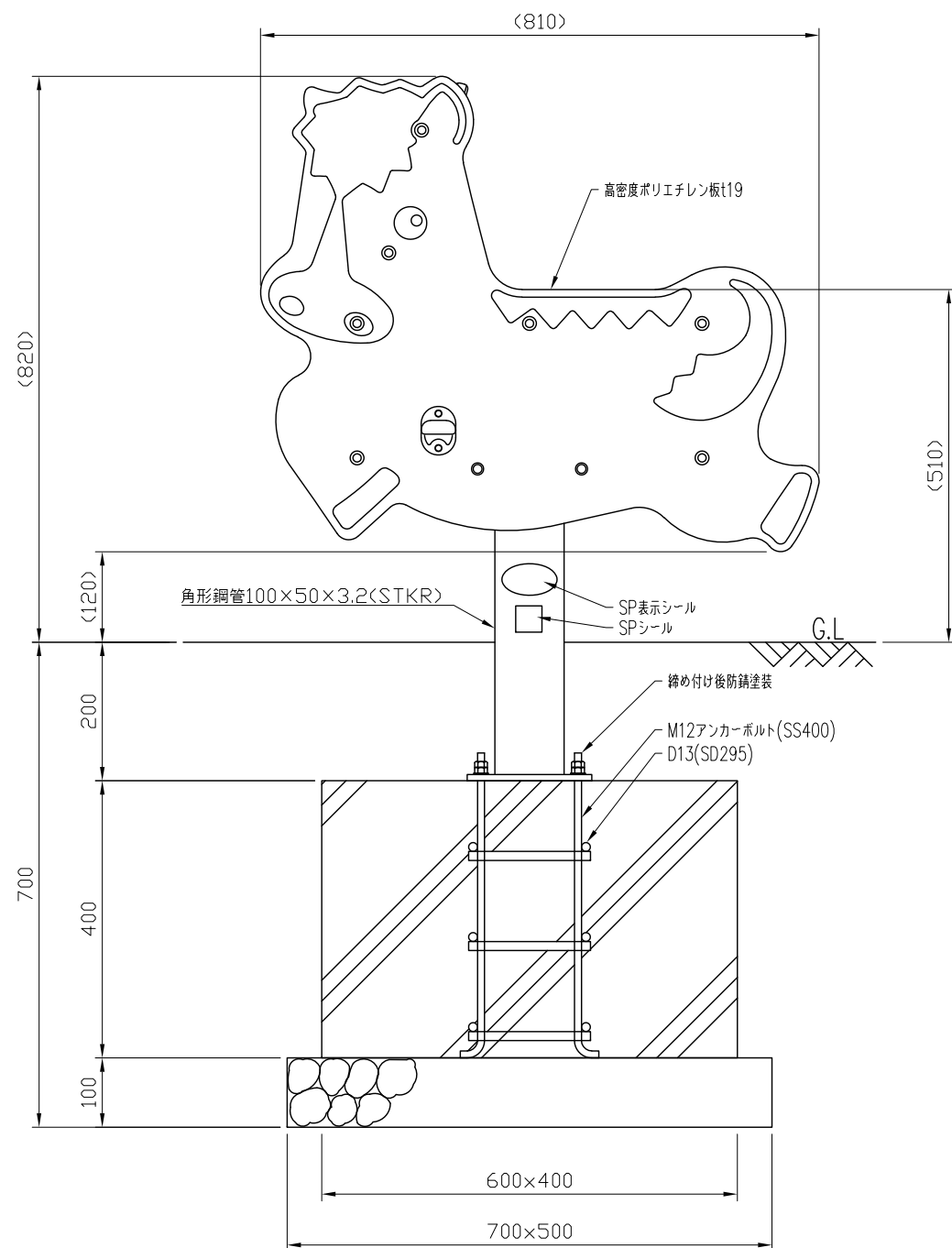
立面図 S=1:10
