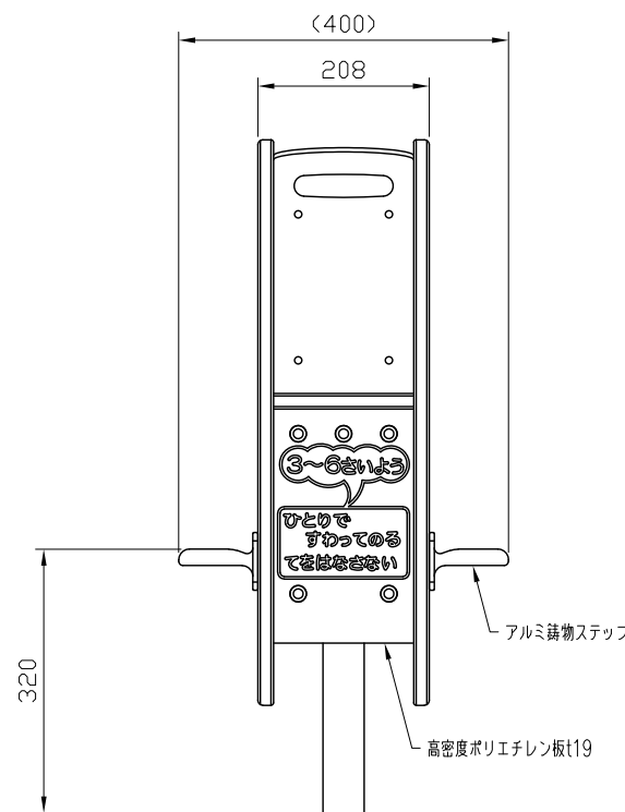
側面図 S=1:10
