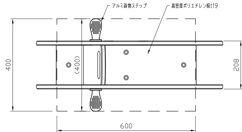
平面図 S=1:10
