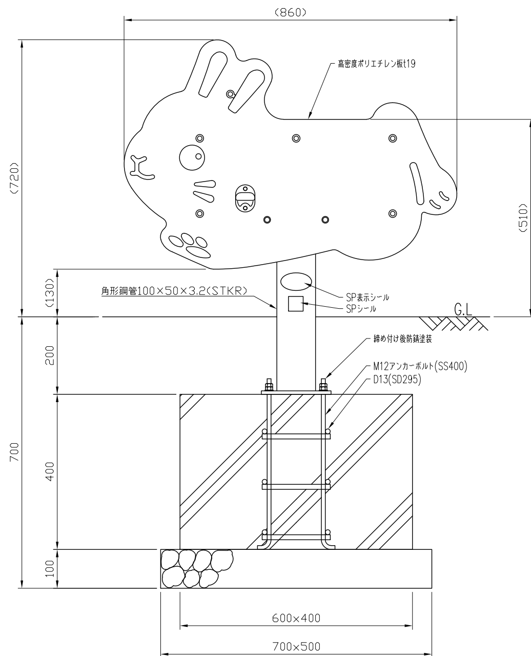
立面図 S=1:10
