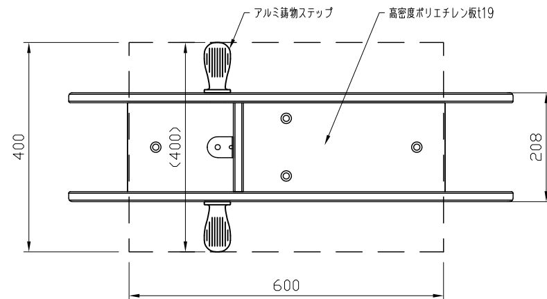
平面図 S=1:10
