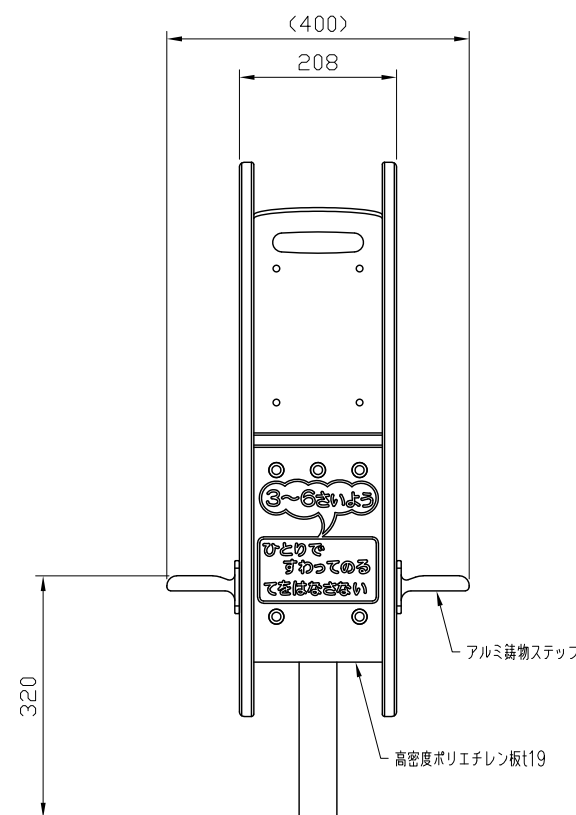
側面図 S=1:10
