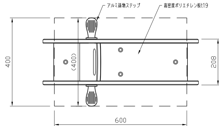
平面図 S=1:10
