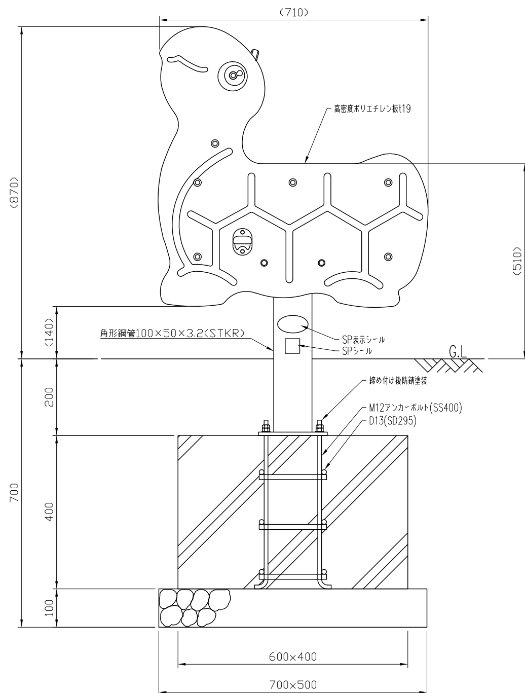
立面図 S=1:10
