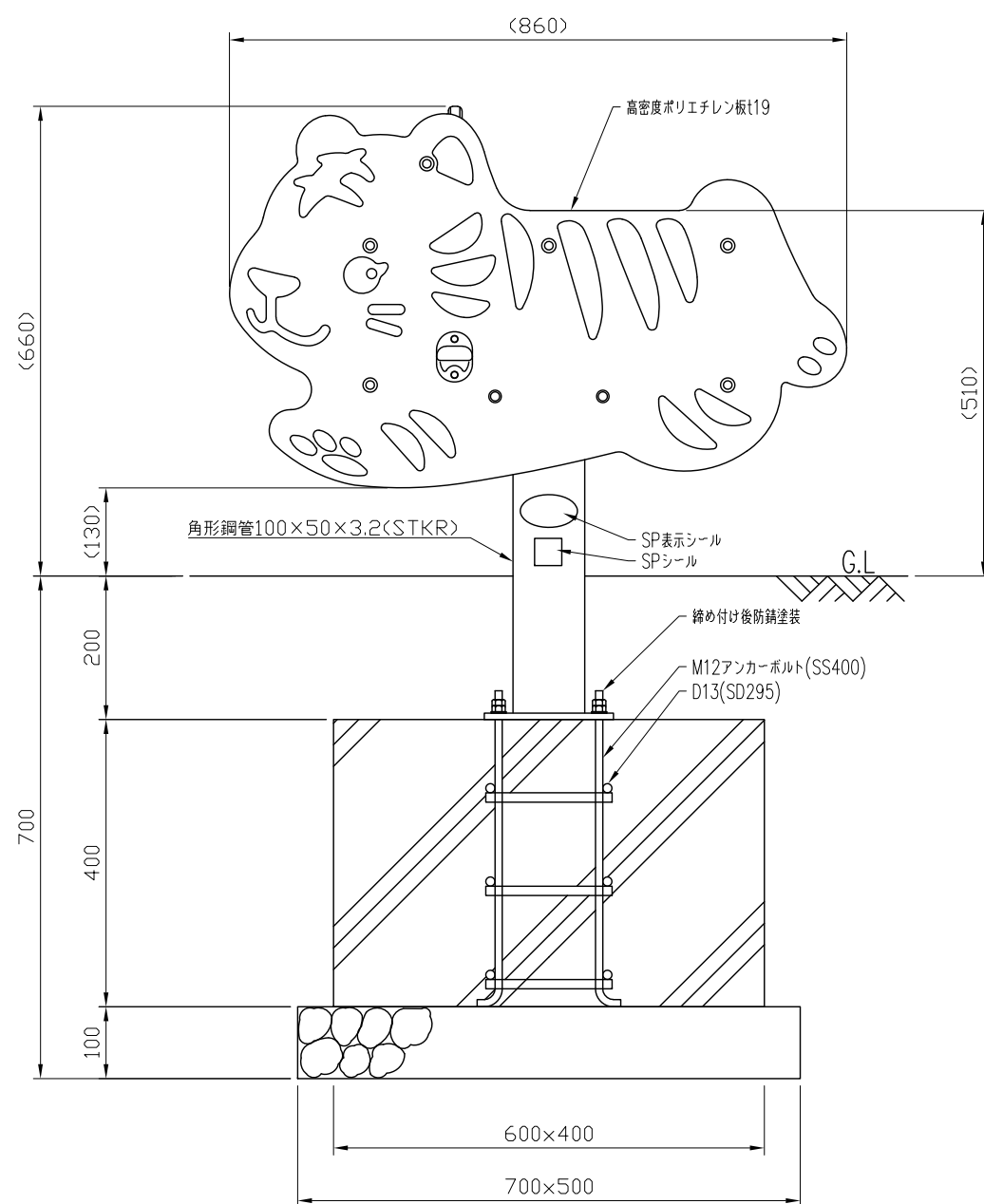
立面図 S=1:10
