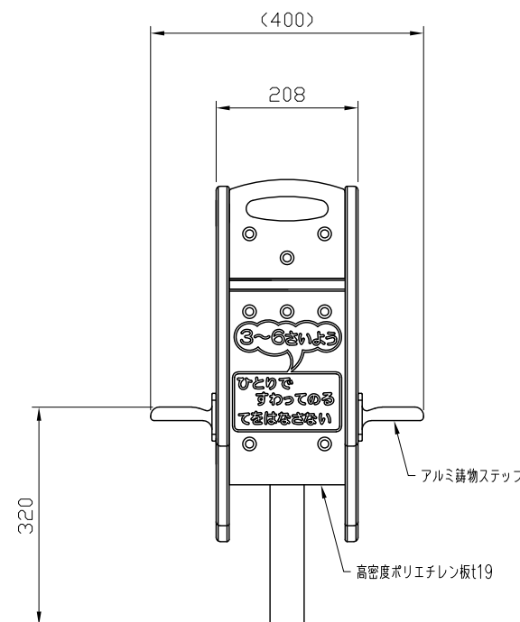
側面図 S=1:10
