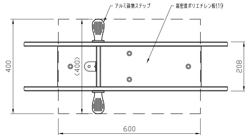
平面図 S=1:10
