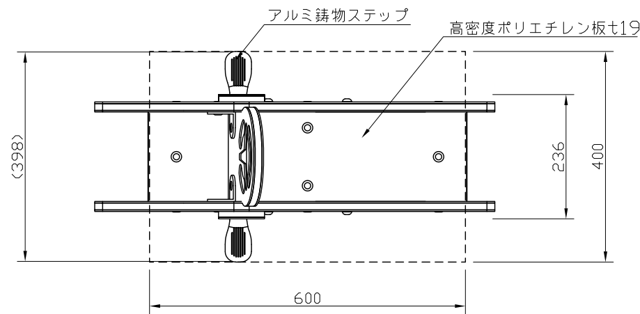
平面図 S=1:10
