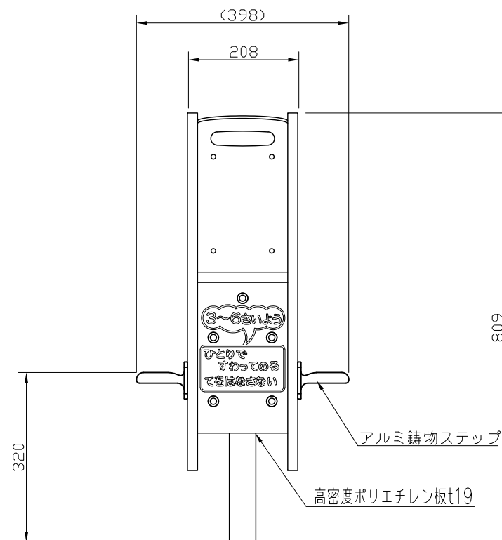
正面図 S=1:10
