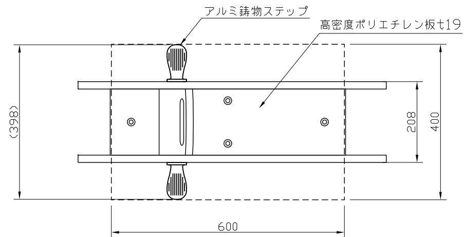
平面図 S=1:10
