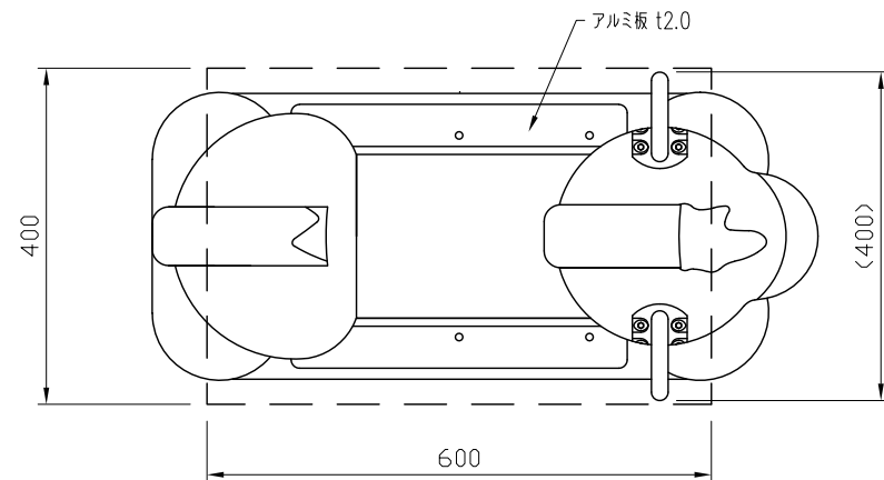
平面図 S=1:10
