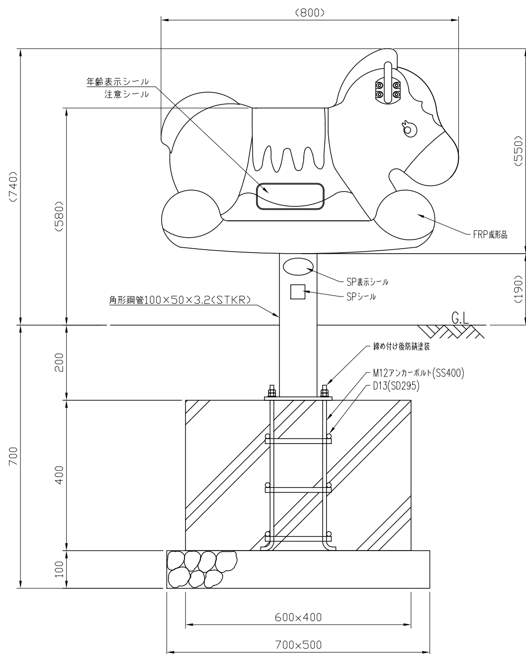
立面図 S=1:10
