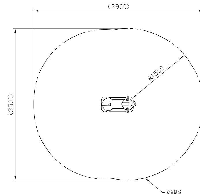
安全領域平面図 S=1:50
