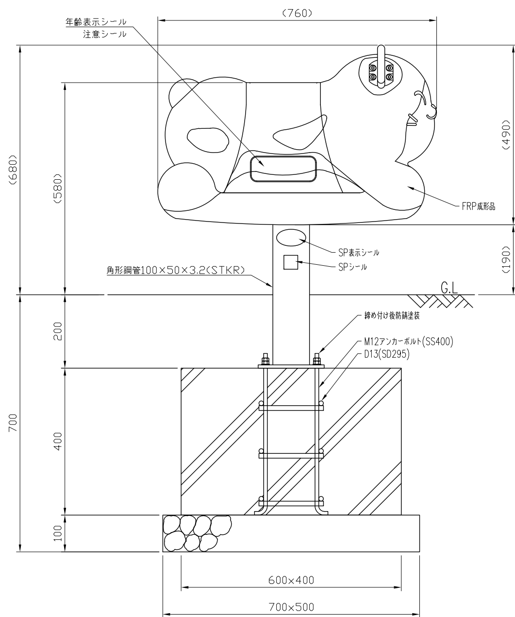
立面図 S=1:10
