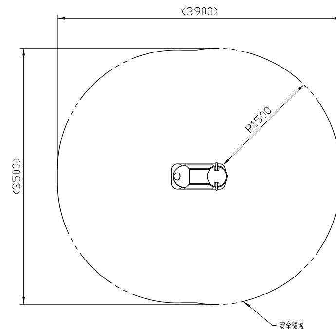
安全領域平面図 S=1:50
