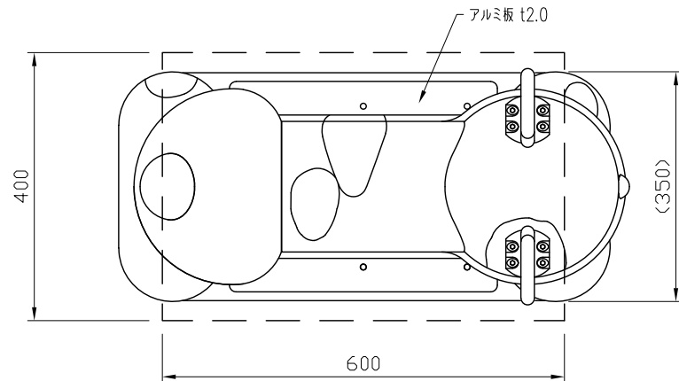
平面図 S=1:10
