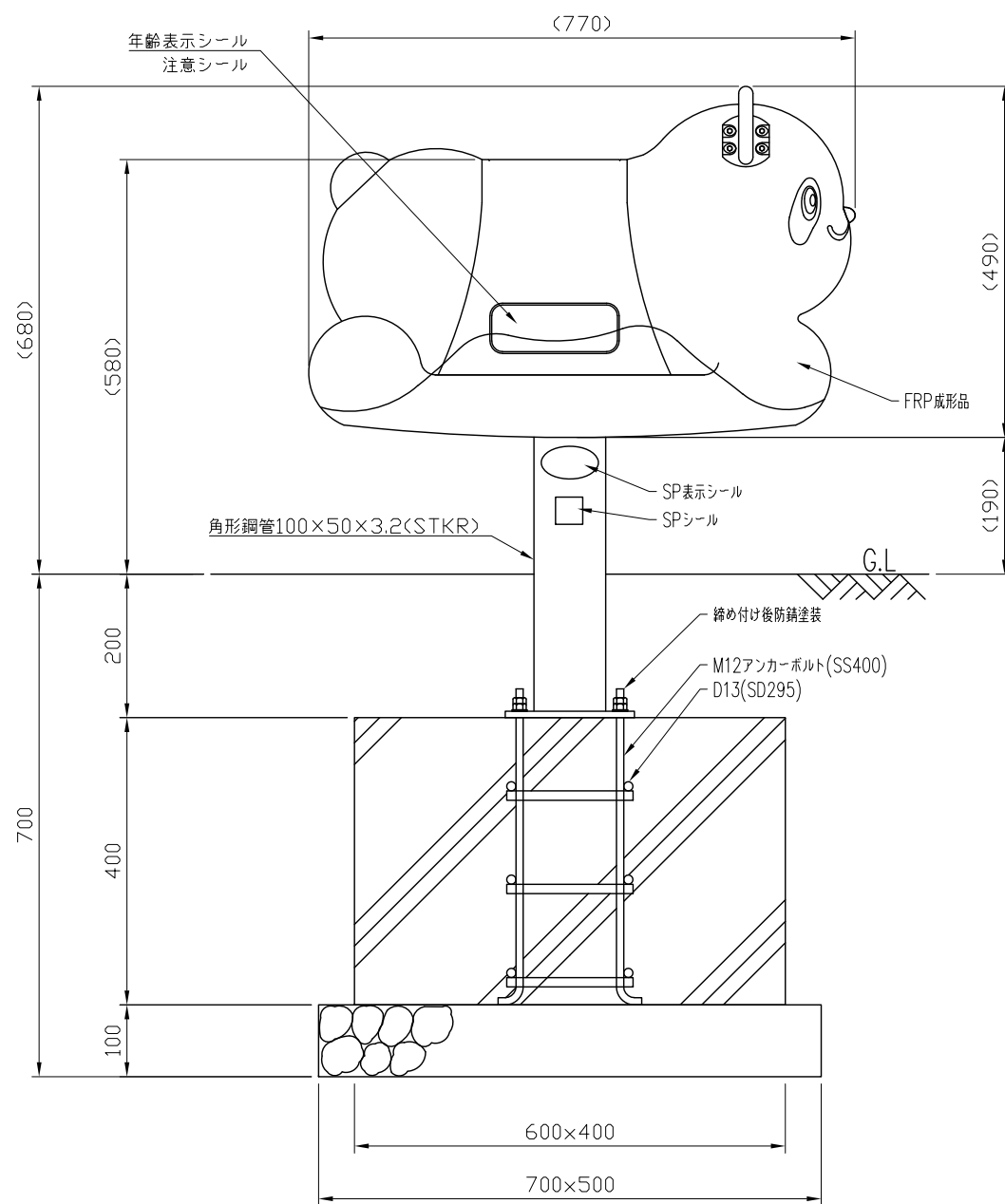
立面図 S=1:10
