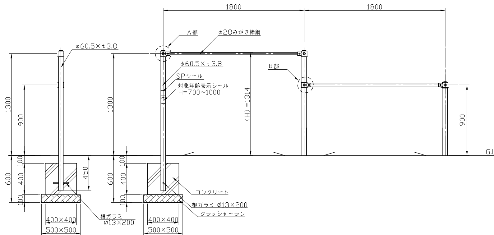
側面図 S=1:30
