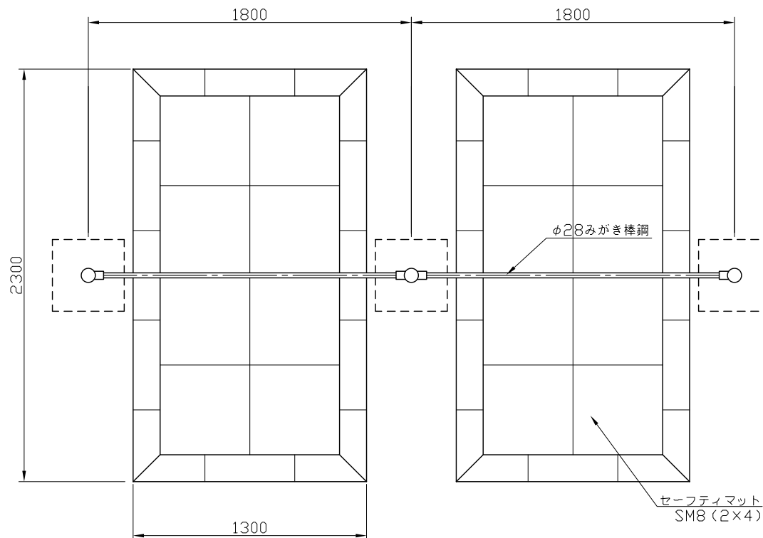
平面図 S=1:30
