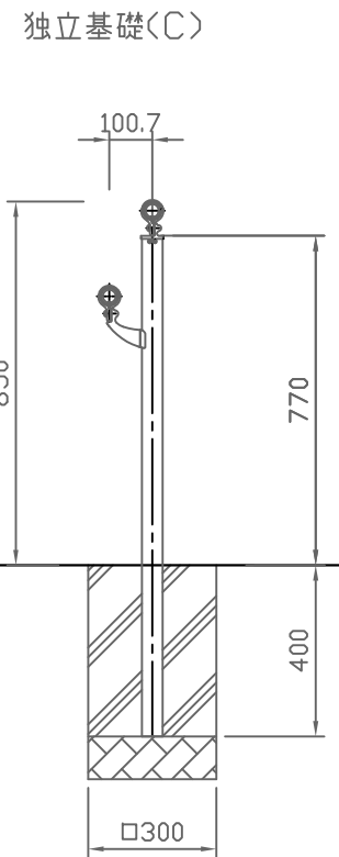
断面図 S=1:20
