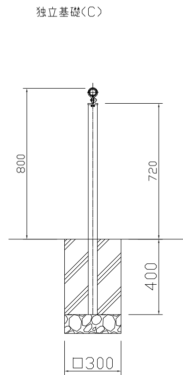
断面図 S=1:20
