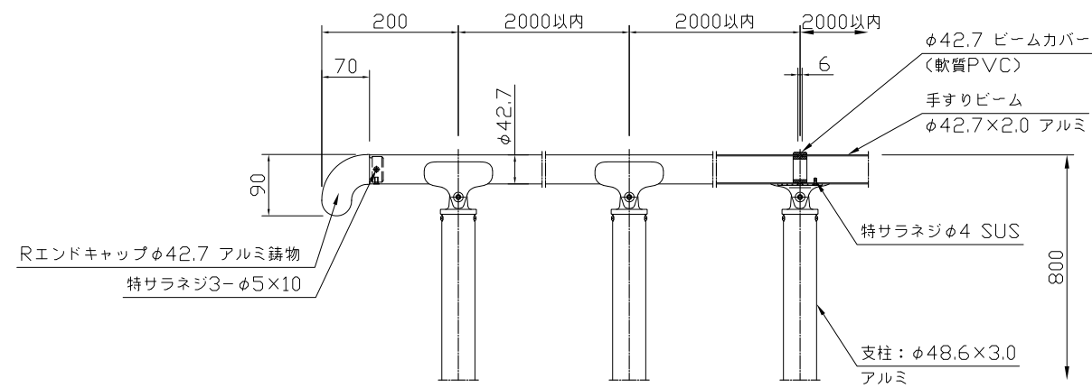
組立詳細図 S=1:10
