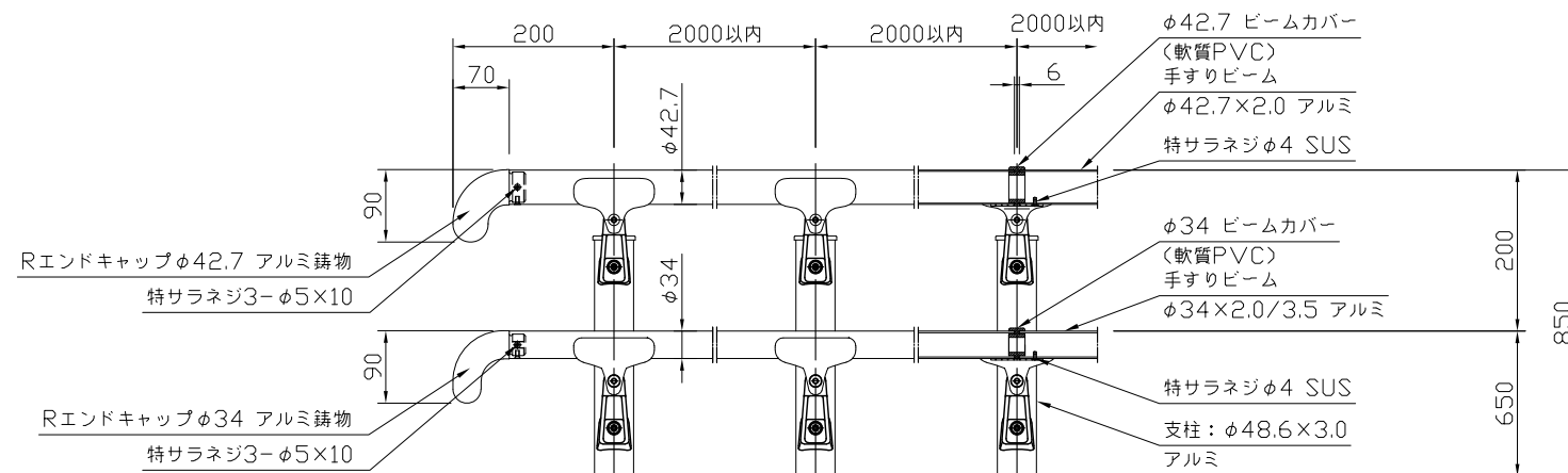
組立詳細図 S=1:10
