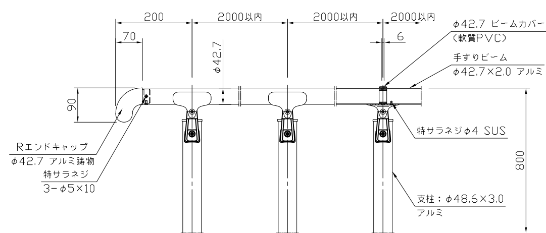
組立詳細図 S=1:10
