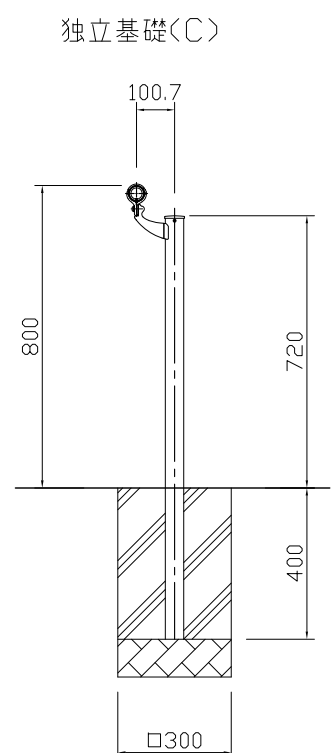
断面図 S=1:20
