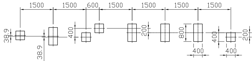
基礎伏図 S=1:100
