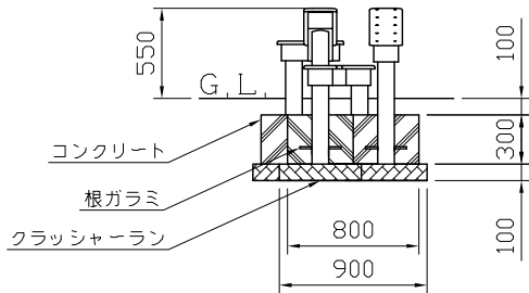
側面図 S=1:50
