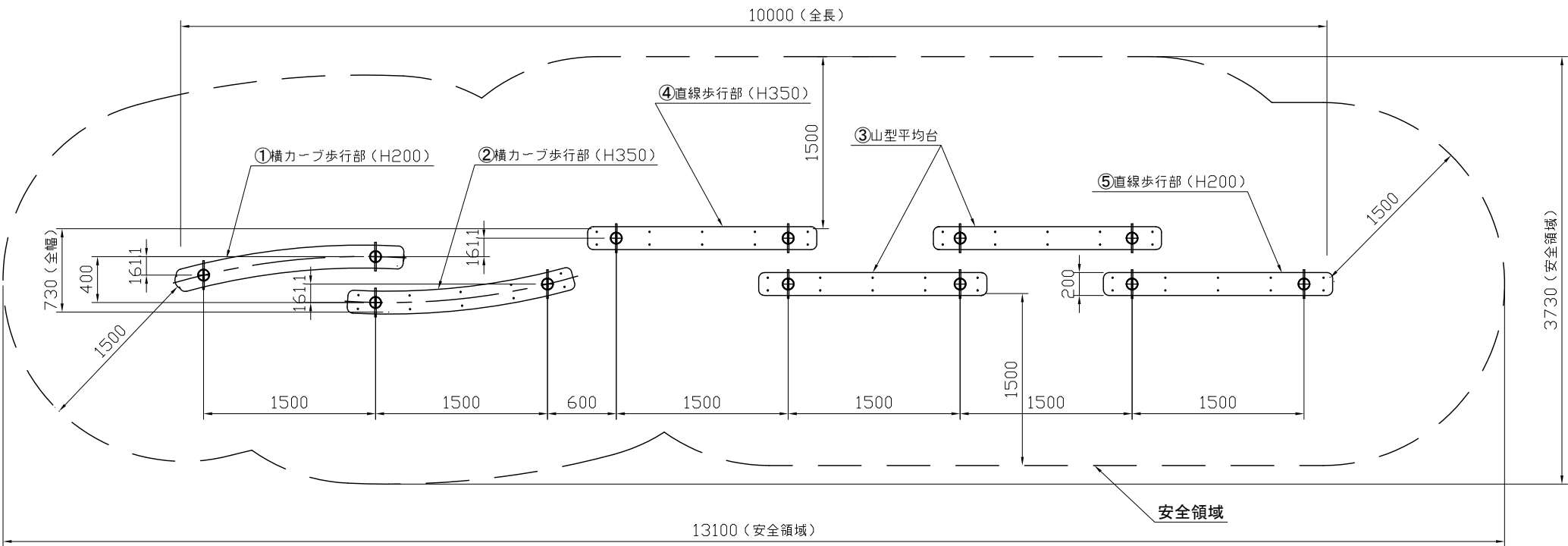
平面図 S=1:50
