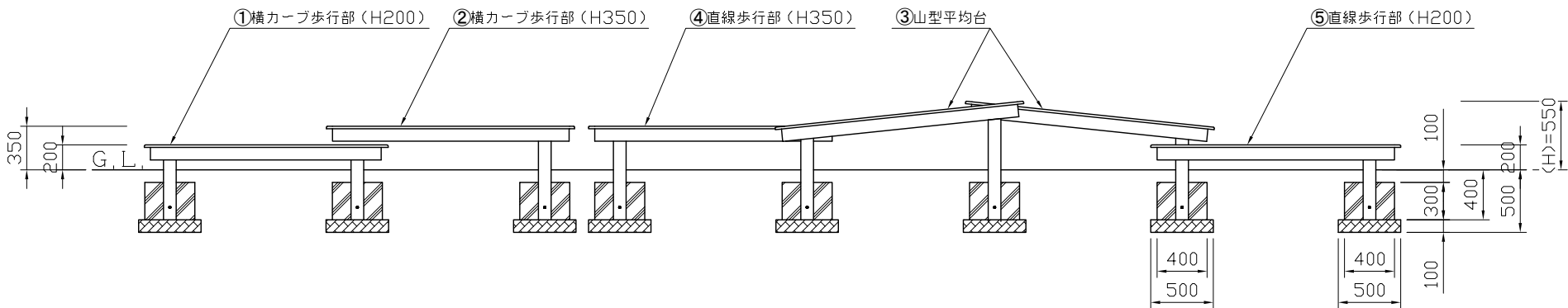
立面図 S=1:50
