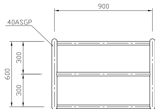
平面図 S=1:20
