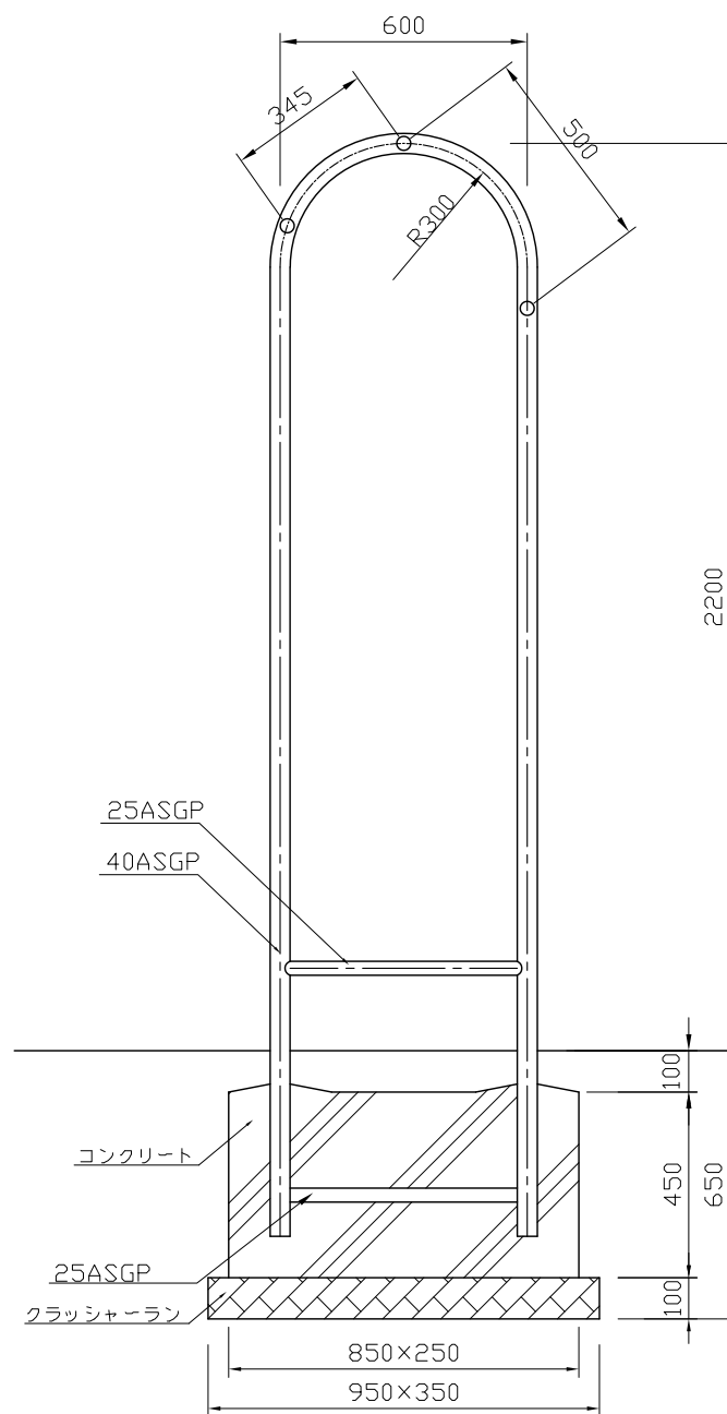
断面図 S=1:20
