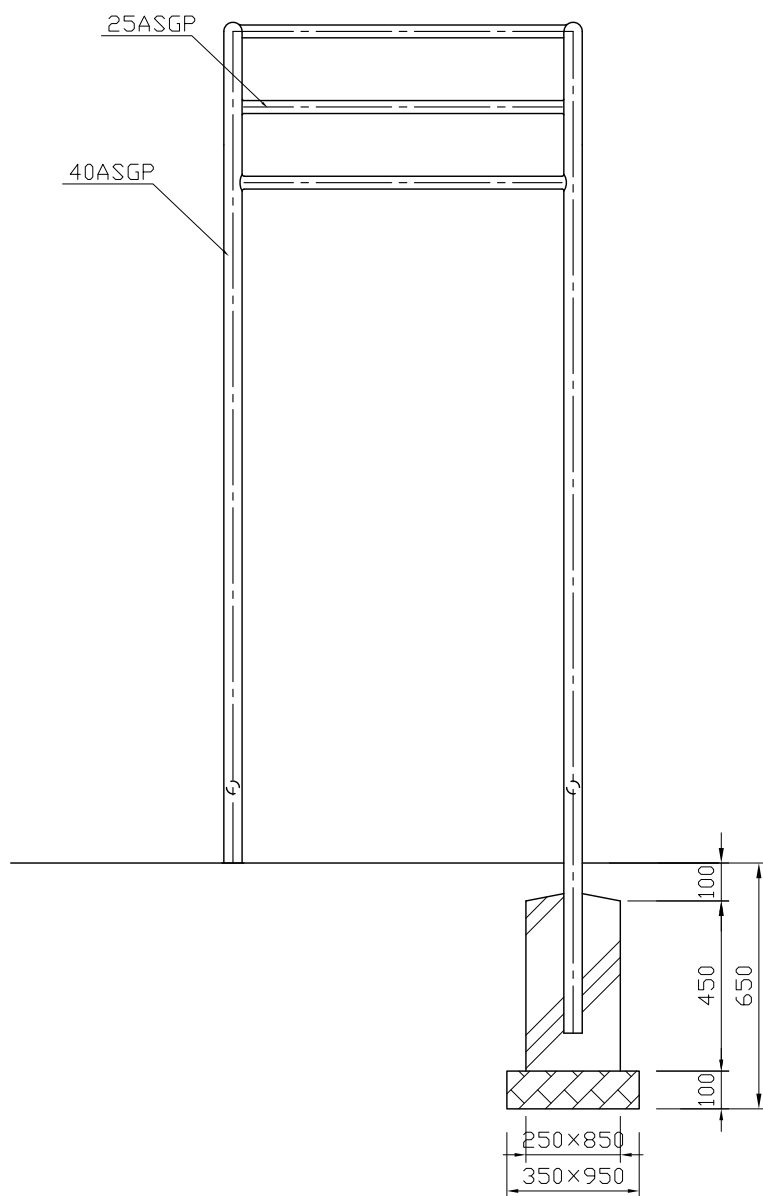
正面図 S=1:20
