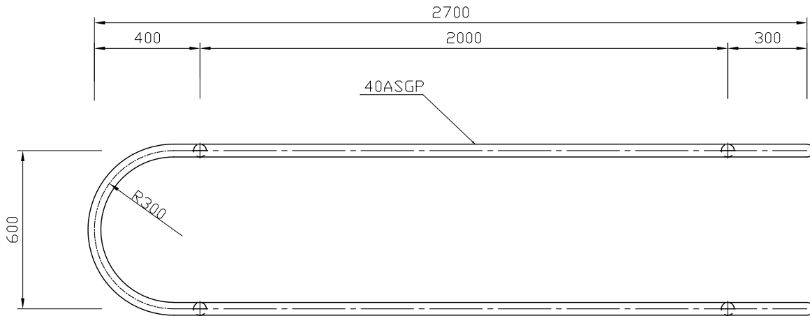
平面図 S=1:20
