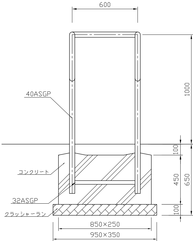
断面図 S=1:20
