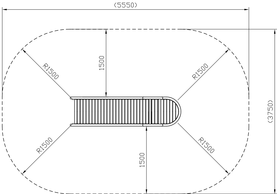
子どもの利用を想定した安全領域平面図 S=1:50
