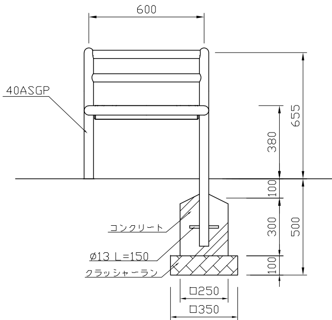
断面図 S=1:20
