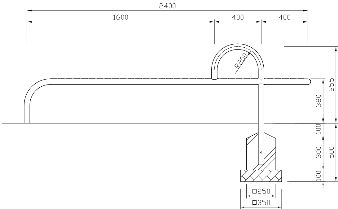
正面図 S=1:20
