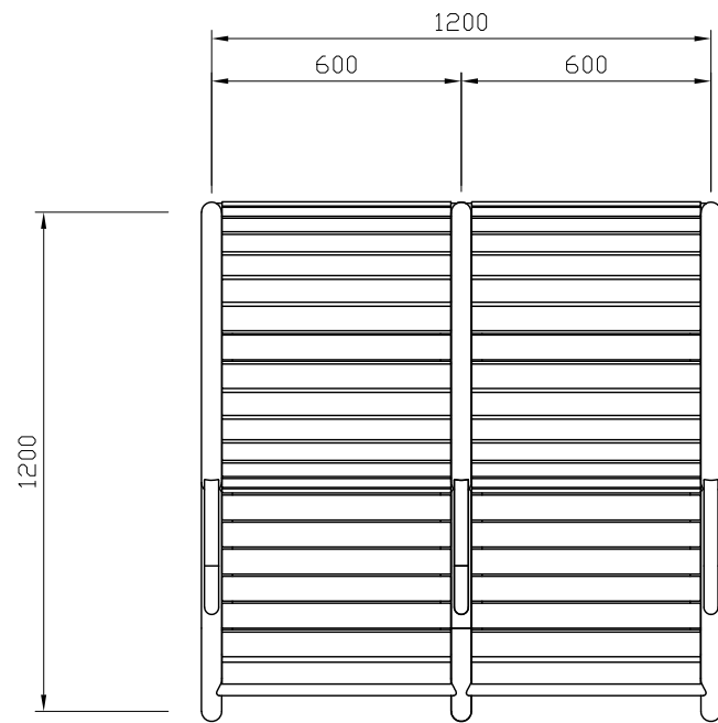
平面図 S=1:20
