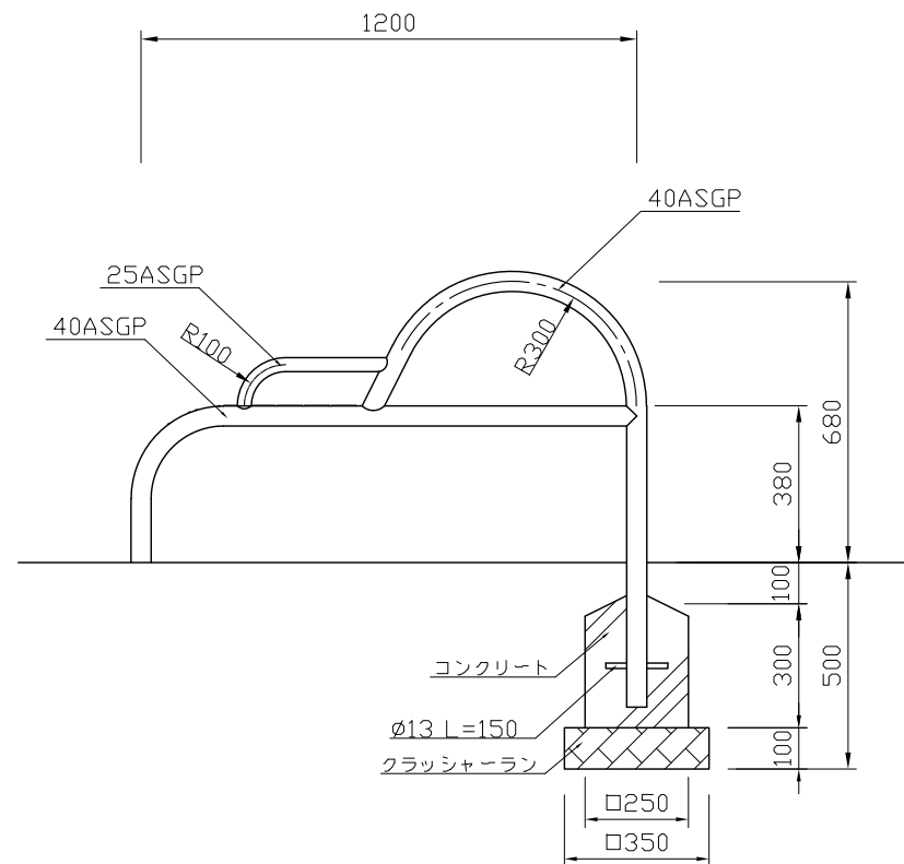
断面図 S=1:20
