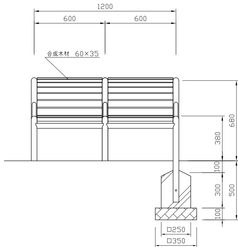
正面図 S=1:20
