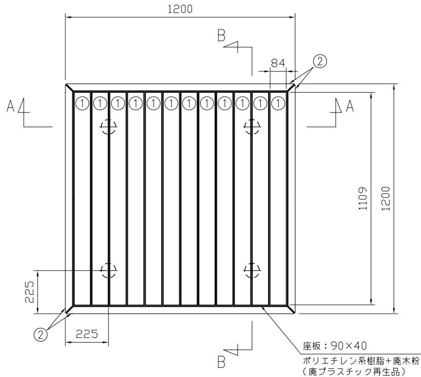
平面図 S=1:20
