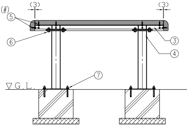
組付断面図(B-B矢視図) S=1:20
