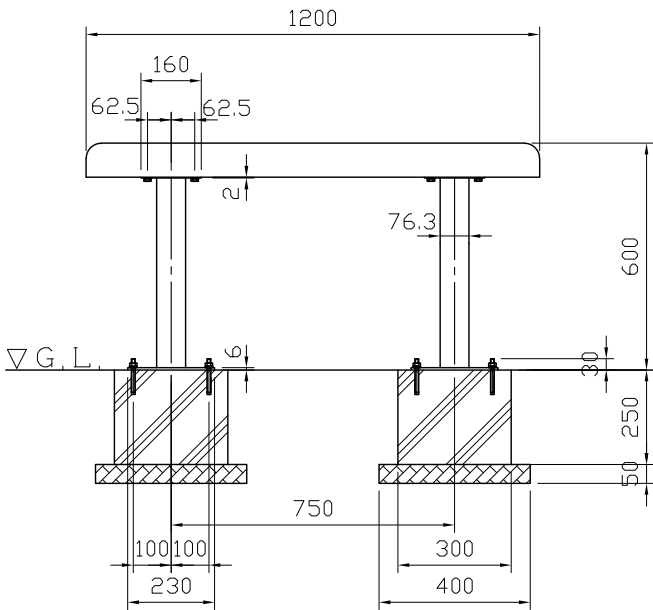
側面図 S=1:20
