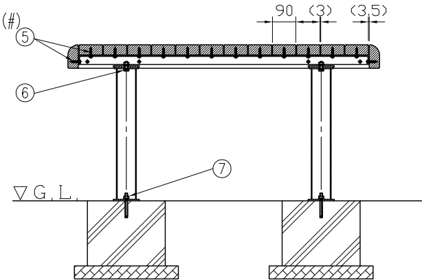
組付断面図(A-A矢視図) S=1:20
