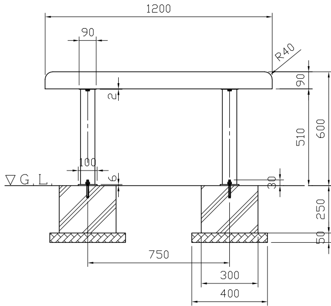
正面図 S=1:20
