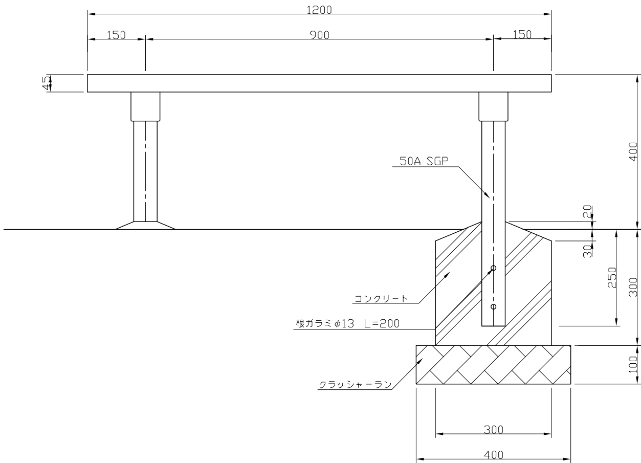
正面図 S=1:10
