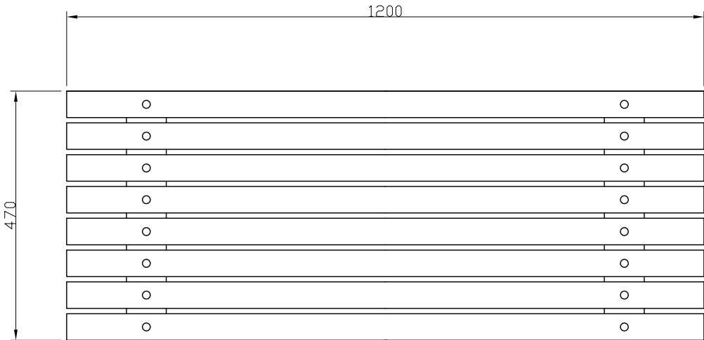
平面図 S=1:10
