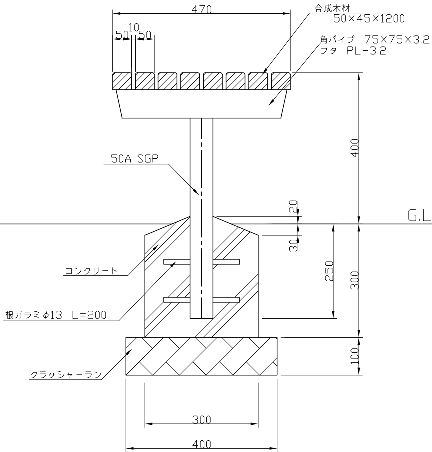
断面図 S=1:10
